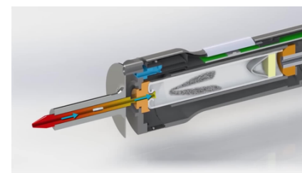
Snap-Vac / принцип работы
